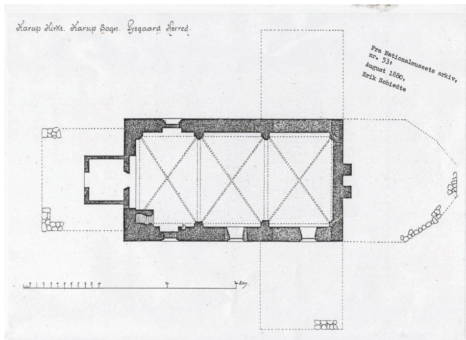
Nationalmuseets tegning over Karup kirkes grundplan. Udført 1880 af dr. Sophus Muller og arkitekt Erik Schiødte
